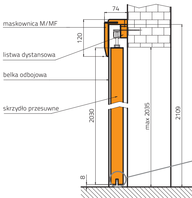
PRZYKŁAD ZASTOSOWANIA SYSTEMU PRZESUWNEGO MOCOWANEGO BEZPOŚREDNIO NA ŚCIANĘ
