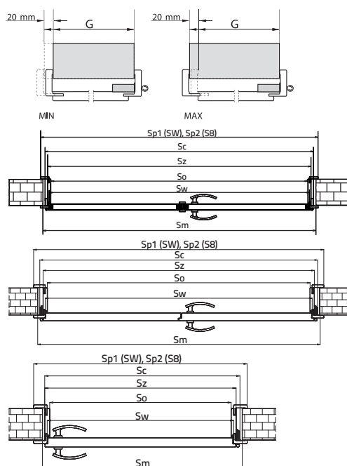
WYMIARY OŚCIEŻNIC REGULOWANYCH SW/S8 DO DRZWI DWUSKRZYDŁOWYCH W TECHNOLOGII STANDARD, SOFT ORAZ TECHNOLOGII RAMA SOFT
