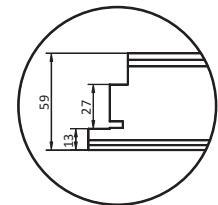
Przekrój skrzydła
