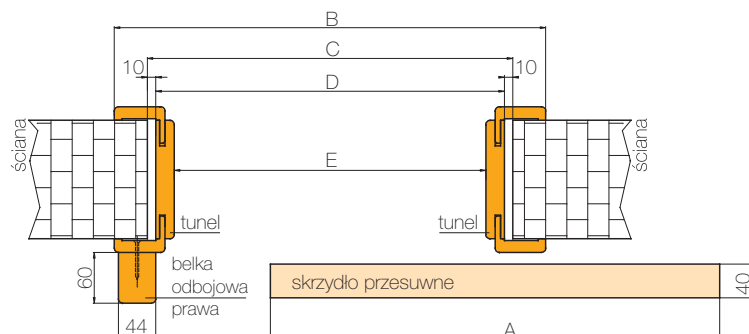
PRZEKRÓJ POZIOMY SYSTEMU PRZESUWNEGO NAŚCIENNEGO Z TUNELEM
